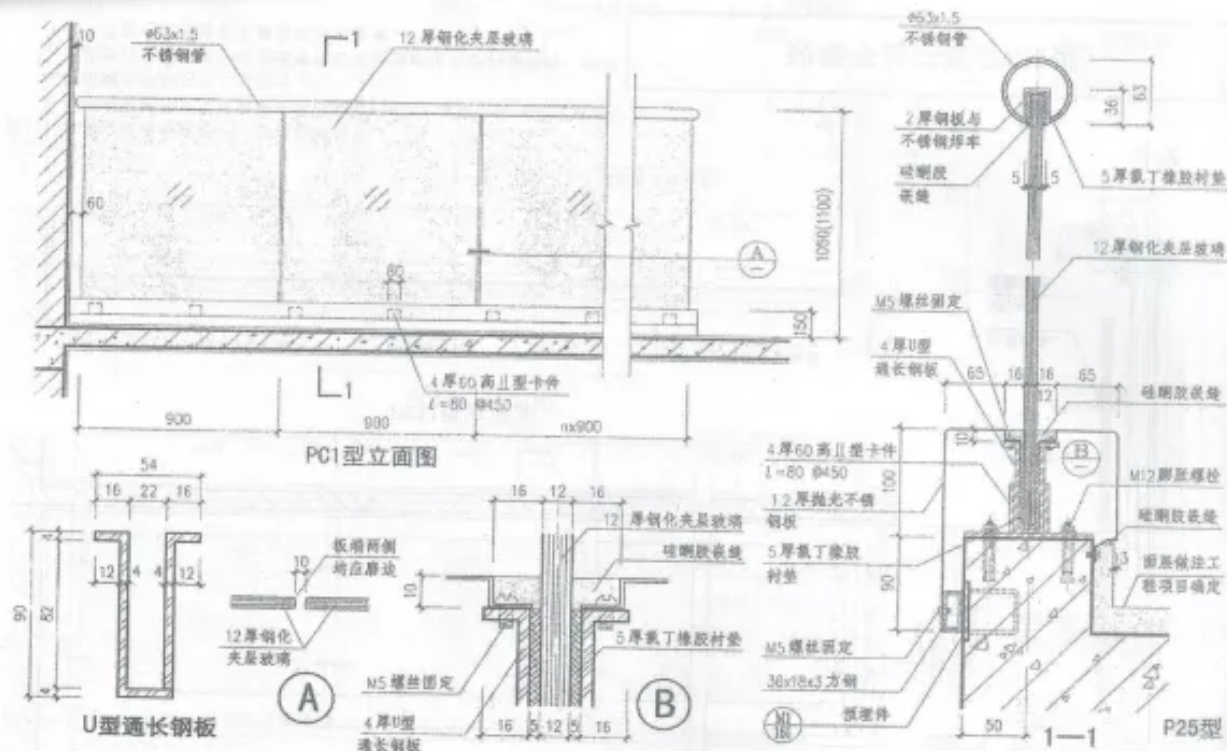
玻璃平台栏杆 (PC1型)
