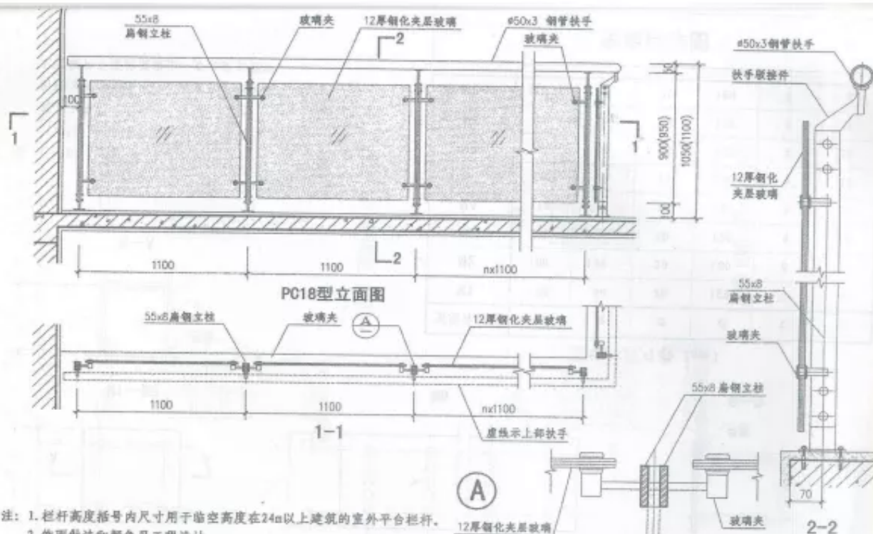
玻璃平台栏杆 (PC18型)
