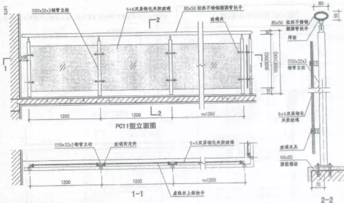
玻璃平台栏杆 (PC11型)
